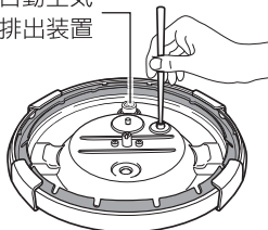
圧力調整弁
